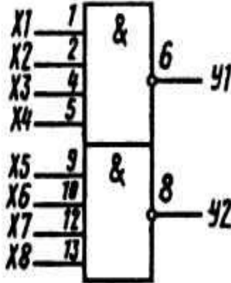
Условное графическое обозначение КР531ЛА16
