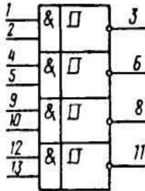
Условное графическое обозначение К155ТЛЗ
