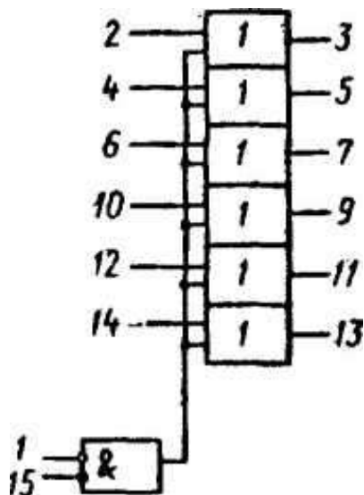
Условное графическое обозначение К155ЛП10
