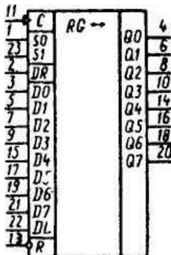
Условное графическое обозначение К155ИР13
