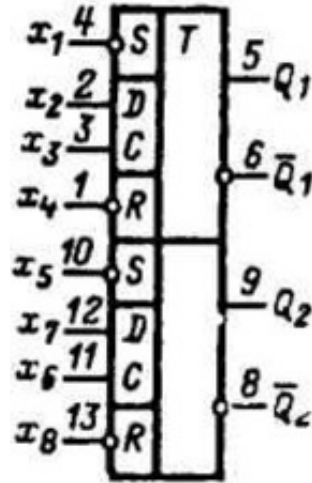
Условное графическое обозначение К131ТМ2
